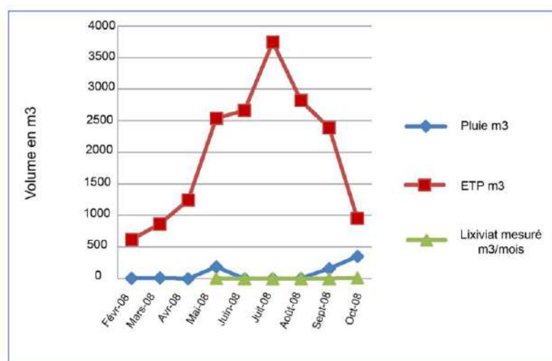
Figure 36: Bilan hydrique sur le casier 2 au CET d'El.Outaya 2008.
