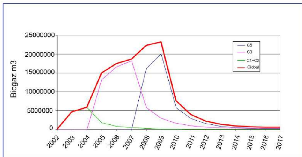
Figure 41 : Production théorique de biogaz en \text{m}^3 \cdot \text{an}^{-1} sur le CET Ouled Fayet.
